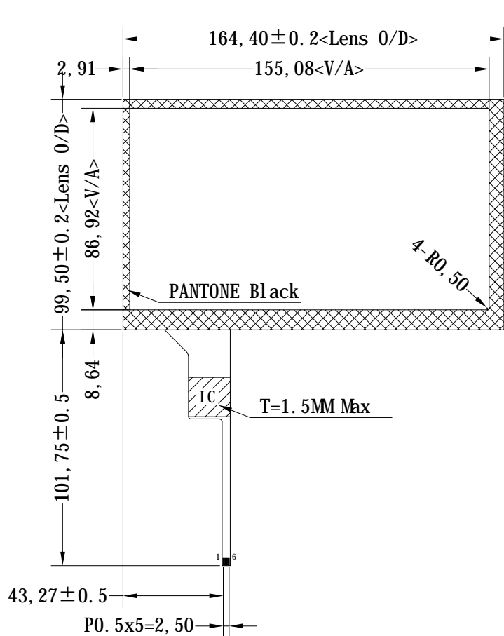
正视图 Front view
