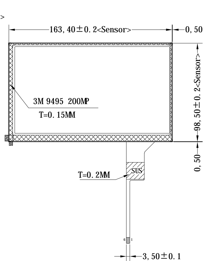
背视图 Back view
